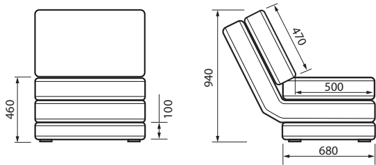
КРЕСЛО 12
