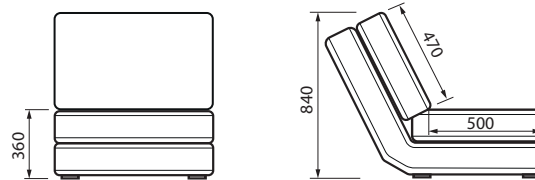
СЕКЦИЯ ОДНОМЕСТНАЯ 10
