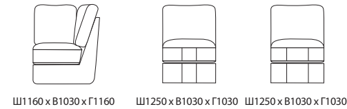
Ш1160 x B1030 x Г1160 Ш1250 x B1030 x Г1030 Ш1250 x B1030 x Г1030
