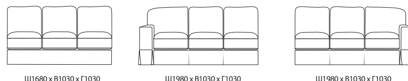
Ш1680 x B1030 x Г1030 Ш1980 x B1030 x Г1030 Ш1980 x B1030 x Г1030
