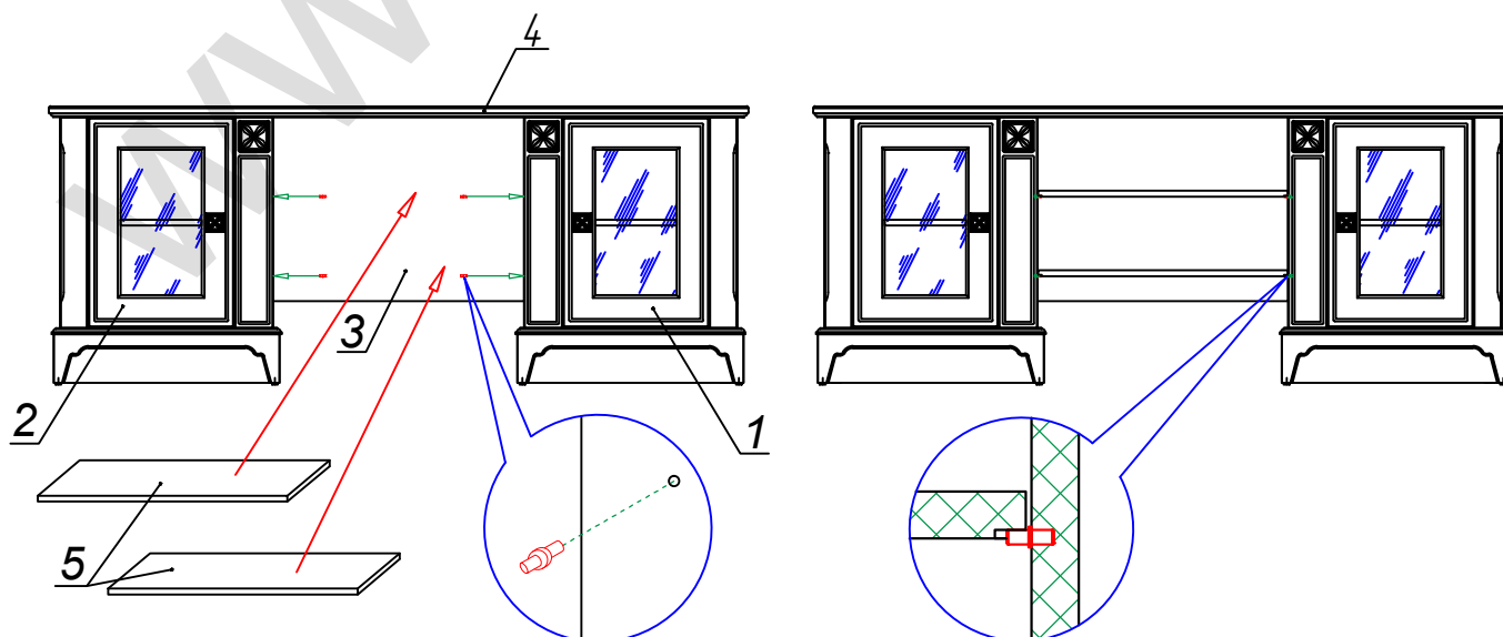
Рис. 4. Схема установки съёмных полок (5)
