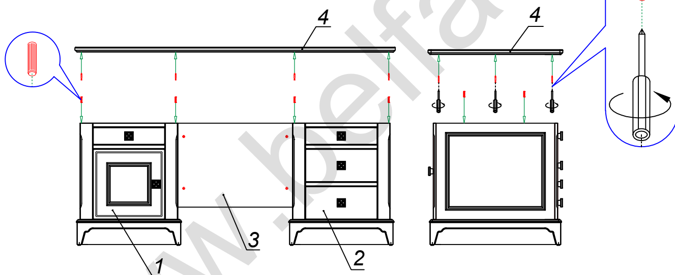
Рис. 3. Схема сборки крышки (4) с тумбами (1) и (2)
