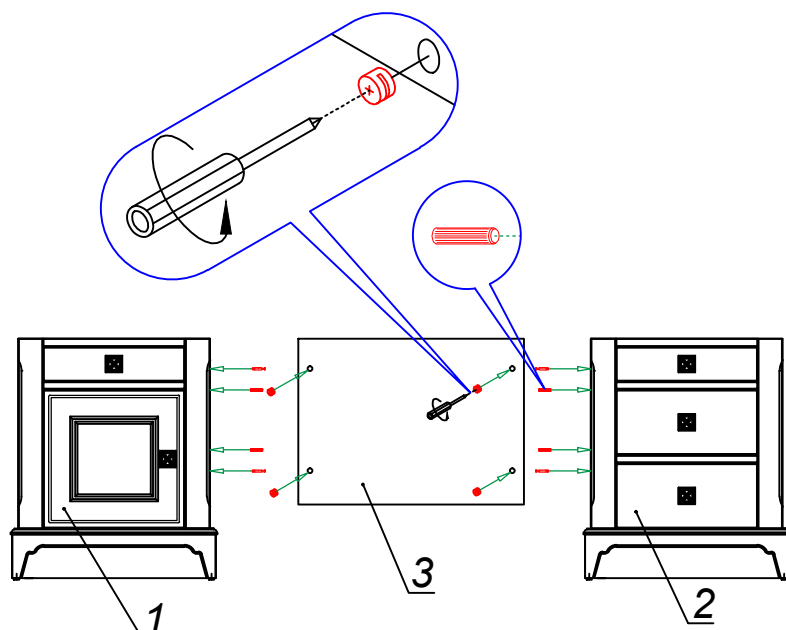
Рис. 2. Схема сборки тумбы левой (1) и тумбы правой (2) со стенкой вертикальной (3)
