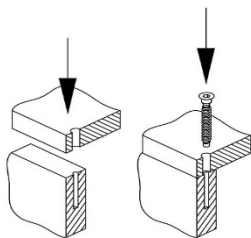
Рис. 5 –Установка винтов-конфирматов
