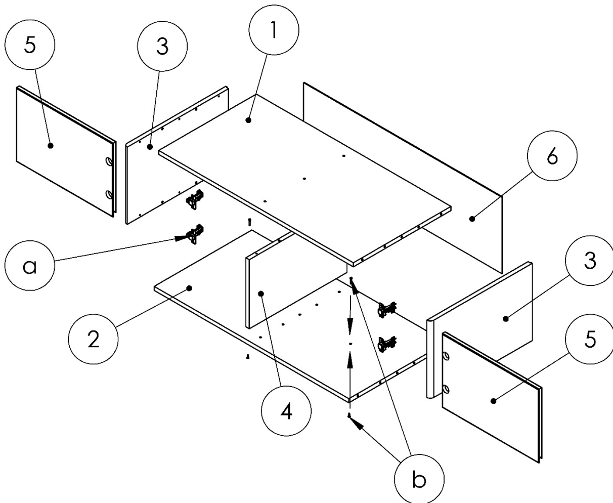
Рис. 2 – Схема сборки
